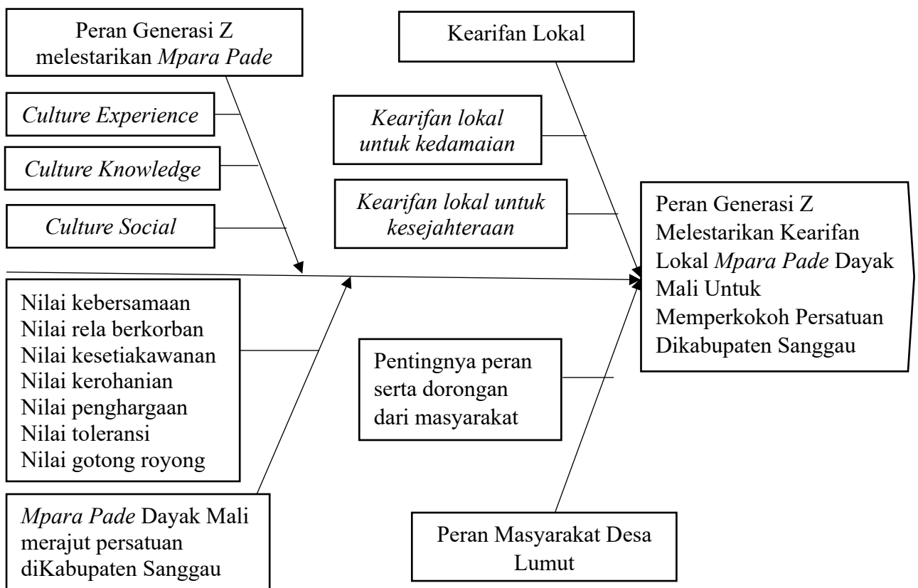
Gambar 2.1 Kerangka Berpikir
